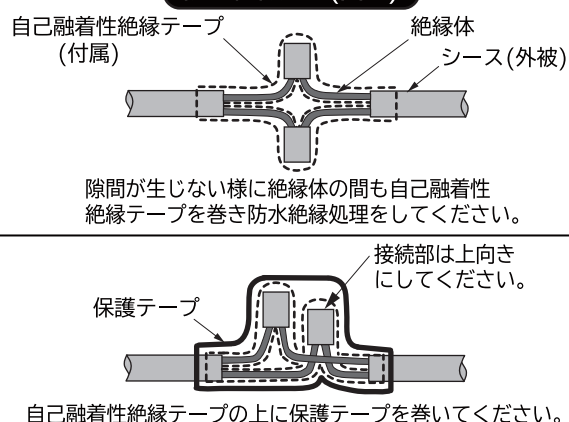
防水絶縁処理(図4)
