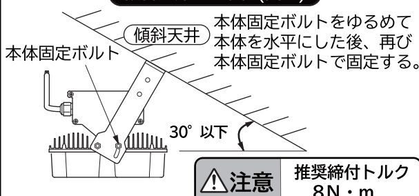
傾斜天井への取付(図3)
