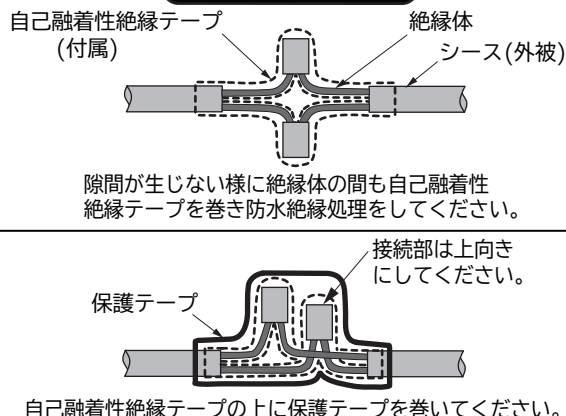
防水絶縁処理(図4)
