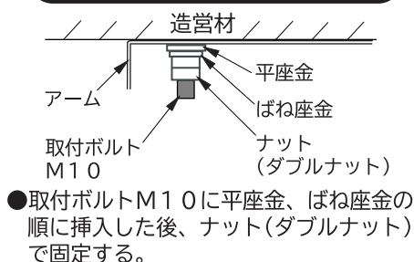
LEDランプの取り付け(図2)
