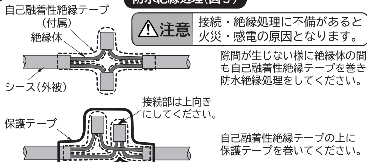
防水絶縁処理(図5)
