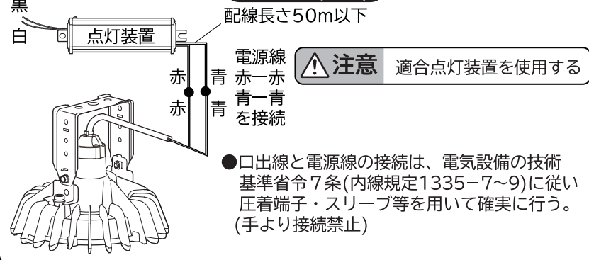
配線接続(図4)
