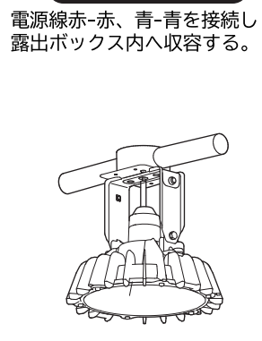
配線接続(図10)
