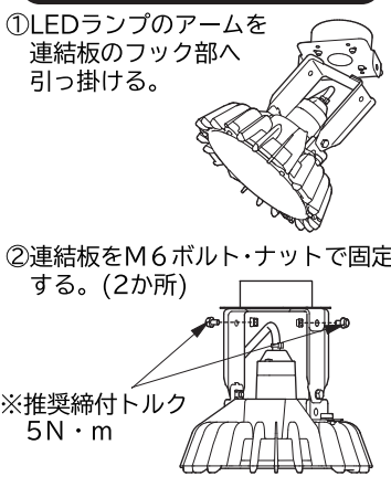
LEDランプの取り付け(図8)
