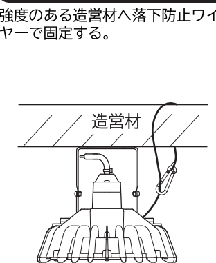
落下防止ワイヤーの取り付け(図9)
