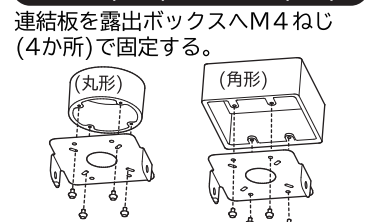
連結板(別売)の取り付け(図7)
