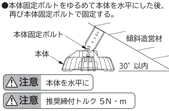
傾斜造営材に取り付ける場合(図5)
