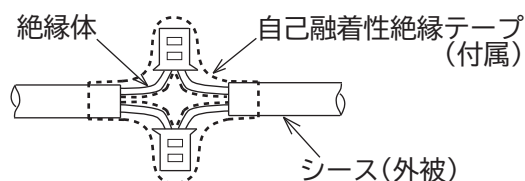
防水絶縁処理 (図3)
