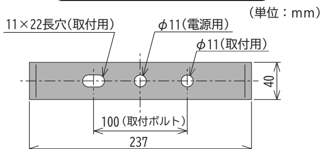
背面取付穴 (図1)
