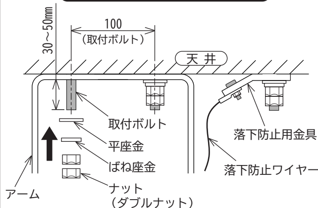
器具取付方法 (図2)
