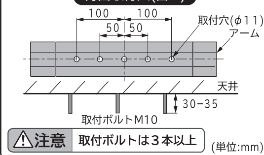
背面取付穴(図1)
