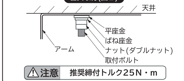
器具取付(図2)
