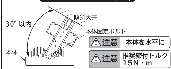
傾斜天井に取り付ける場合(図3)
