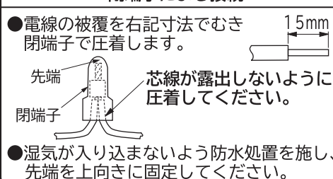
閉端子による接続
