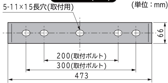
背面取付穴(図1)
