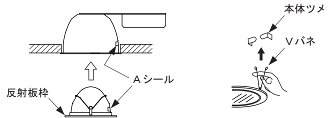
反射板枠取り付け方(図5)
