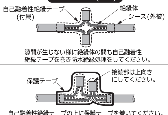
防水絶縁処理(図3)
