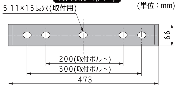
背面取付穴(図1)
