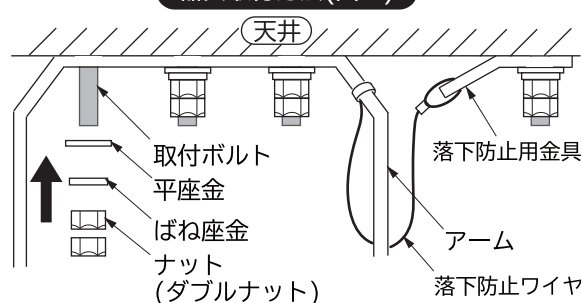
器具取付方法(図2)
