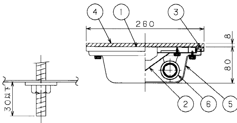
器具内寸法
