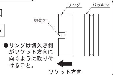
蛍光ランプの取り付けかた（図4）
