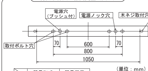
背面取付穴と器具質量(図1)
