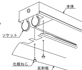
反射板の取り付けかた（図3）
