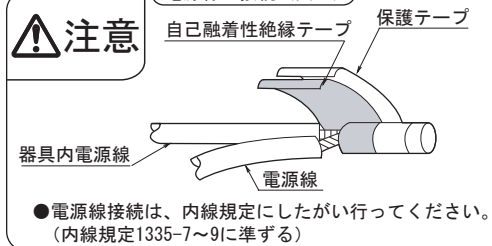
電源線の接続(図2)
