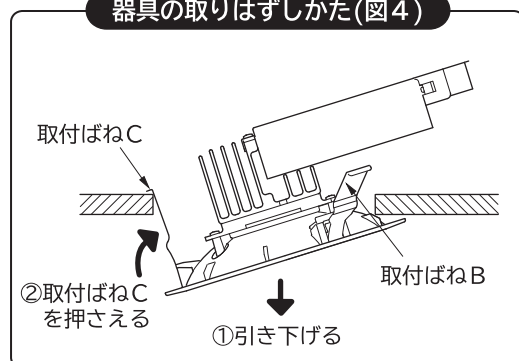
器具の取りはずしかた(図4)
