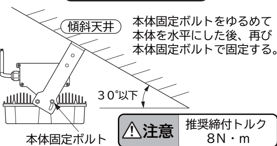
傾斜天井への取付(図3)
