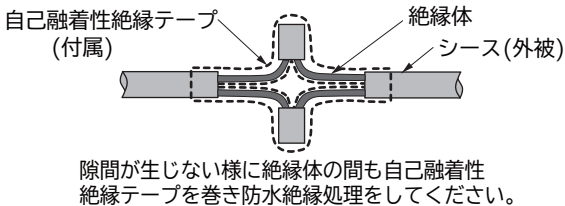
防水絶縁処理(図4)
