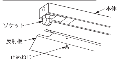
反射板の取り付けかた(図3)
