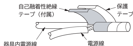
電源線の接続(図2)
