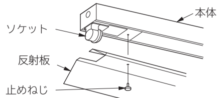
反射板の取り付けかた (図3)
