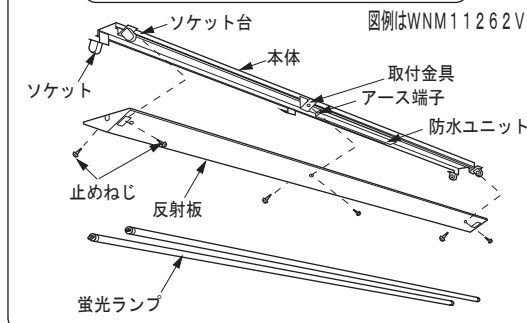
各部の名称(図1)
