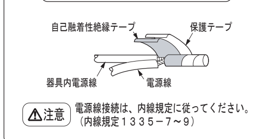
電源線接続のしかた(図5)
