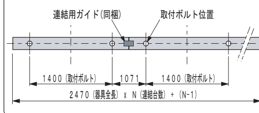
単体N連結する場合の取付ピッチ(図3)
