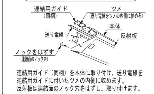
連結のしかた(図4)
