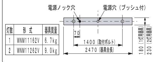
器具質量と背面取付穴(図2)
