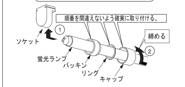
ソケットキャップの取り付けかた(図6)
