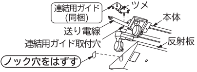
電源線の接続(図3)
