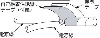
電源線の接続(図3)
