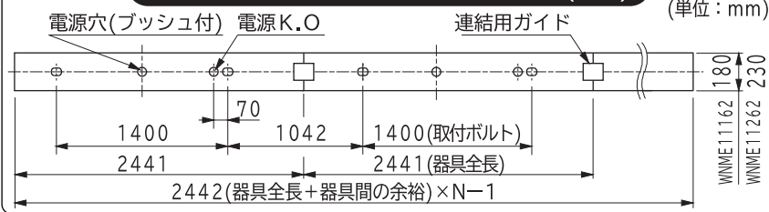
単体N台連結で使用する場合の取付ピッチ(図1)
