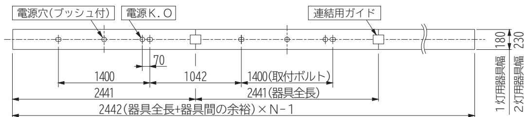
単体N台連結で使用する場合の取付ピッチ (図1)
