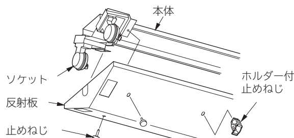
反射板の取り付けかた (図4)
