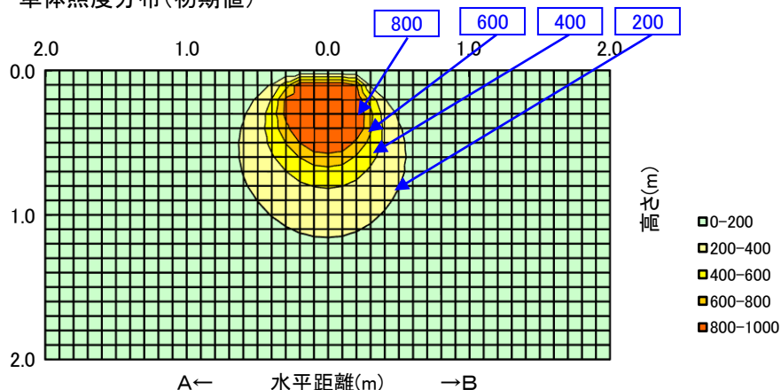
单体照度分布(初期値)
