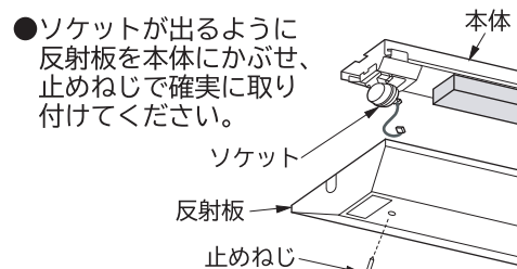
反射板の取り付けかた(図3)
