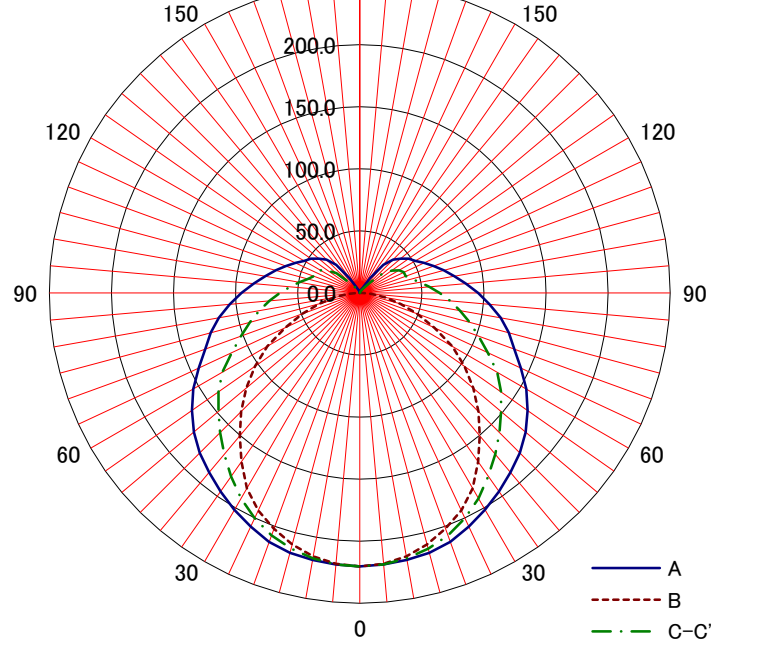
配光曲線 (cd/1000 lm)
