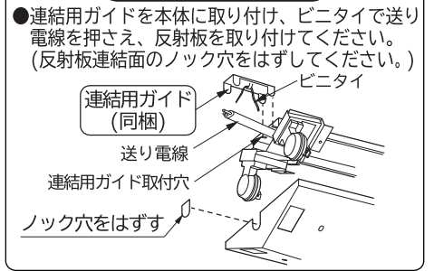
電源線の接続(図3)
