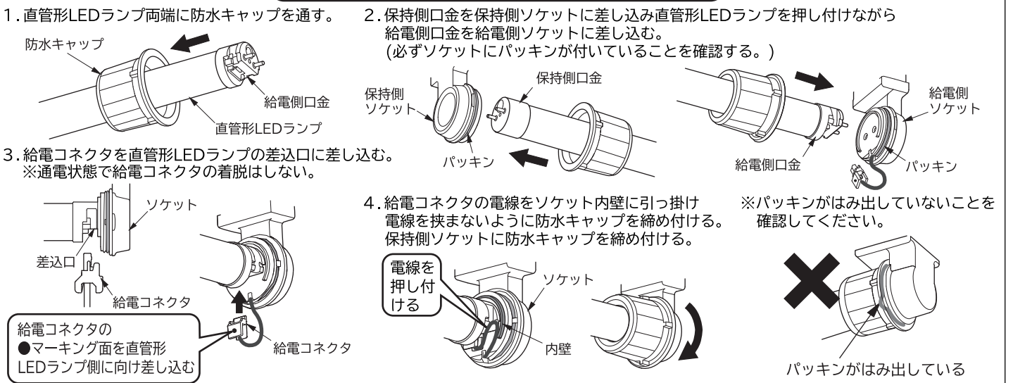
直管形LEDランプと防水キャップの取り付けかた(図5)
