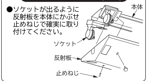
反射板の取り付けかた(図4)
