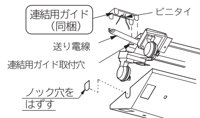
電源線の接続(図3)
