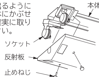
反射板の取り付けかた(図4)
