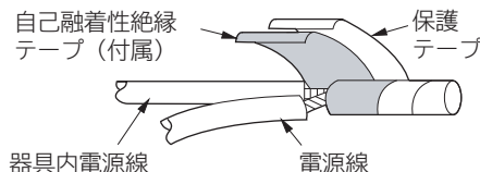
電源線の接続(図3)
