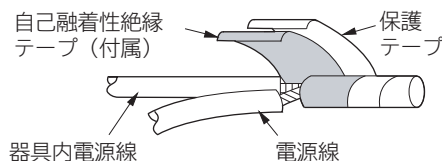
電源線の接続 (図2)
