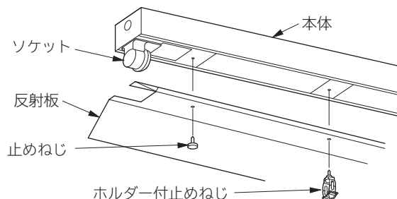
反射板の取り付けかた (図3)
