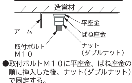
LEDランプの取り付け(図2)
