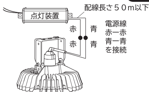
配線接続(図4)
