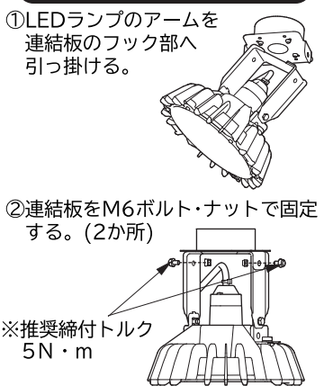
LEDランプの取り付け(図8)
