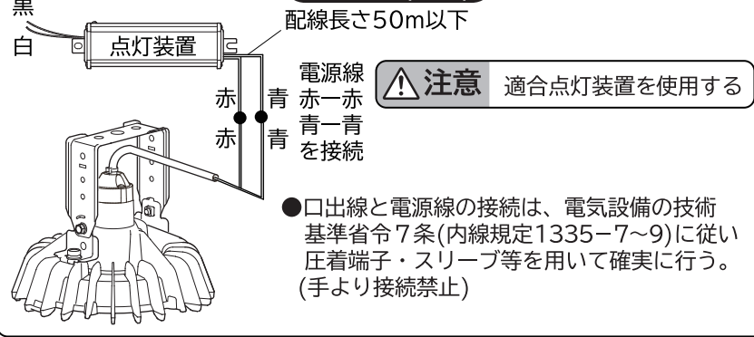
配線接続(図4)
