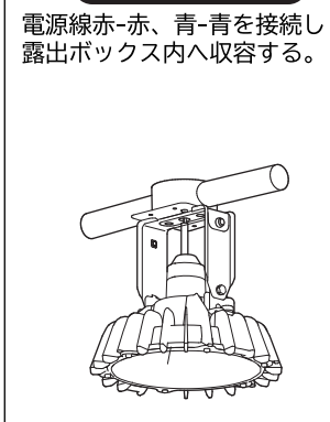
配線接続(図10)
