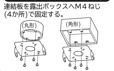
連結板(別売)の取り付け(図7)
