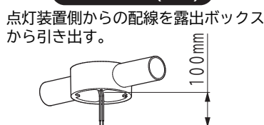
連結板(別売)の取り付け(図7)
