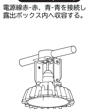
配線接続(図10)
