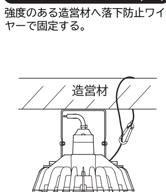
落下防止ワイヤーの取り付け(図9)
