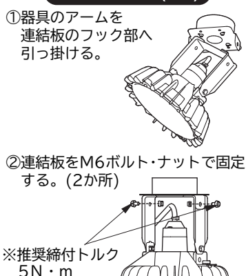
器具の取り付け(図8)
