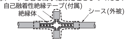
防水絶縁処理(図11)
