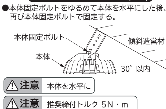
傾斜造営材に取り付ける場合(図5)
