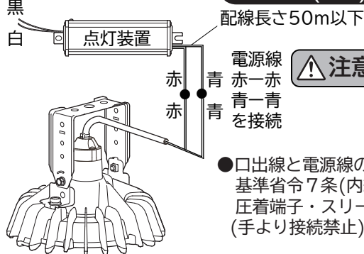
配線接続(図4)
