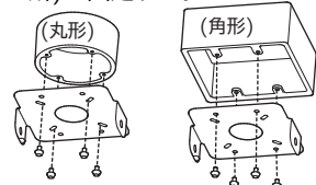
連結板(別売)の取り付け(図7)
