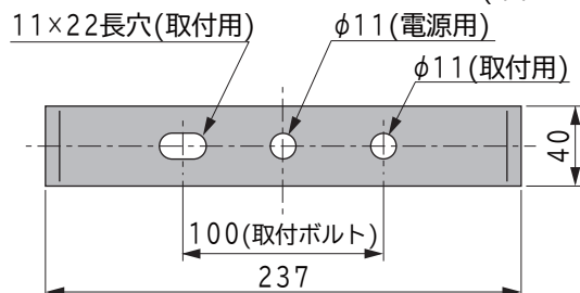
器具取付方法(図2)
