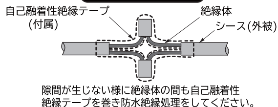
防水絶縁処理(図4)
