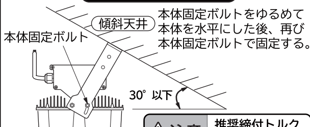
傾斜天井への取付(図3)
