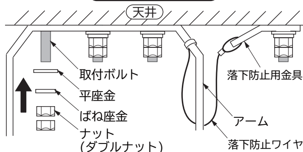
器具取付方法(図2)
