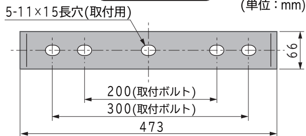
背面取付穴(図1)
