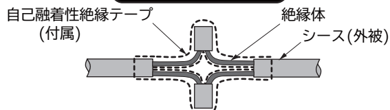
防水絶縁処理(図4)
