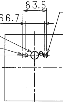
取付寸法図
