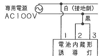
遠隔操作を使用しない結線
