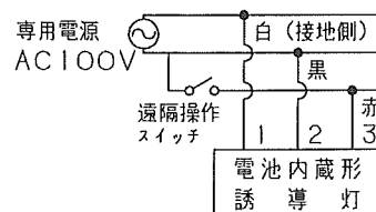
遠隔操作を使用する結線
