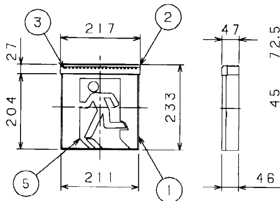
背面取付図
