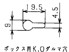
ボックス用K.O.穴
