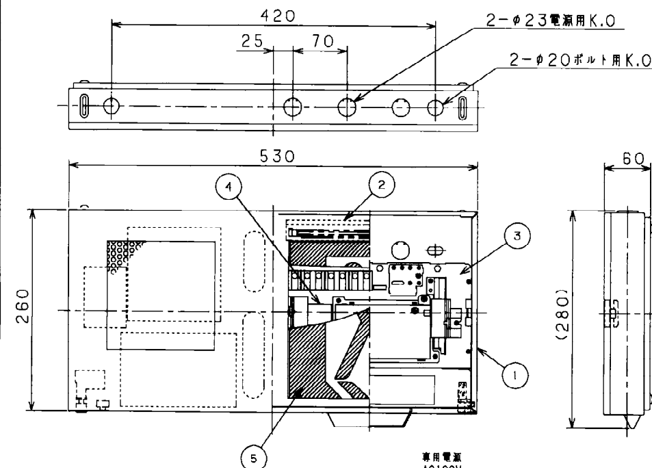
取付寸法図
