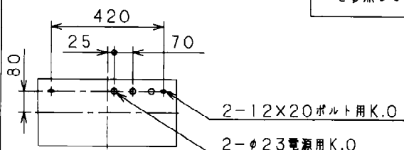
取付寸法図
