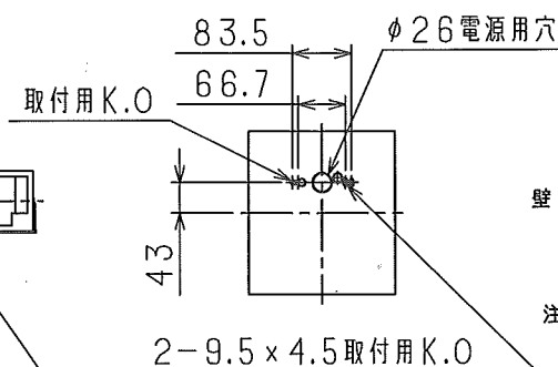
取付寸法図
