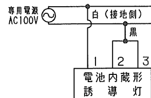
遠隔操作を使用しない結線
