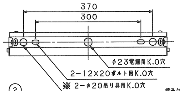
インサートボルト(器具取付ボルト) 器具内寸法
