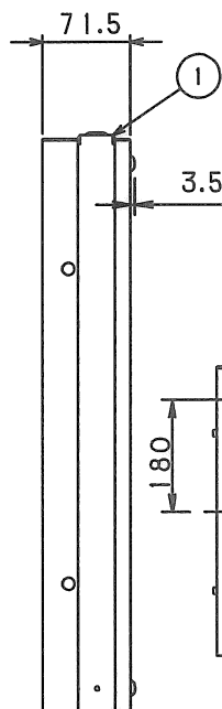
背面取付図
