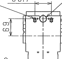
取付寸法図
