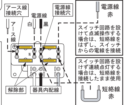
端子台の電流容量20A
