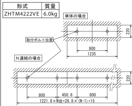
天井埋込穴 (図 1)
