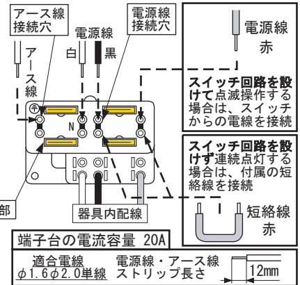
蓄電池の接続 (図 4)
