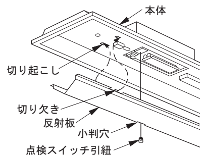
反射板の取り付け (図 5)
