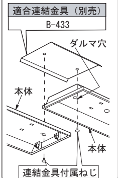
連結のしかた (図 2)
