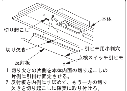
反射板の取り付け (図5)
