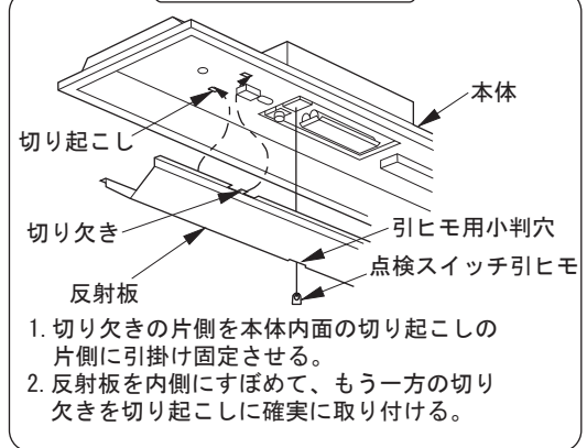
反射板の取り付け (図5)
