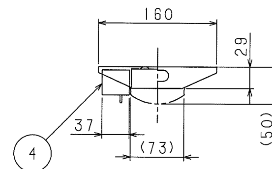
側面詳細図
