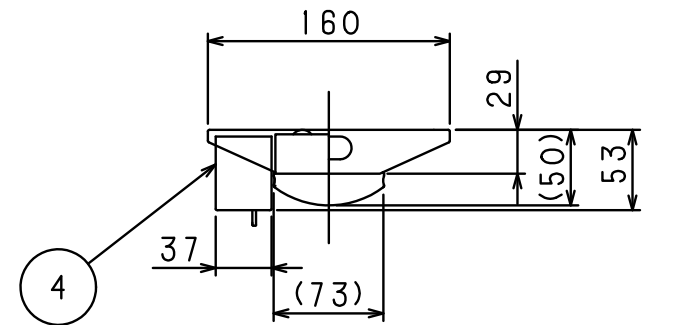
側面詳細図
