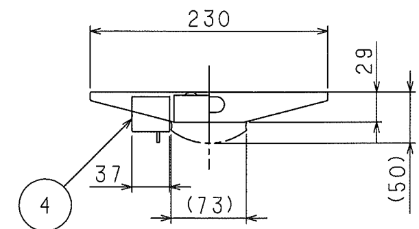
側面詳細図
