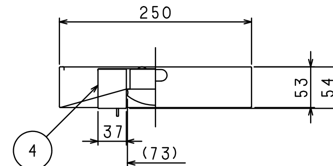
側面詳細図
