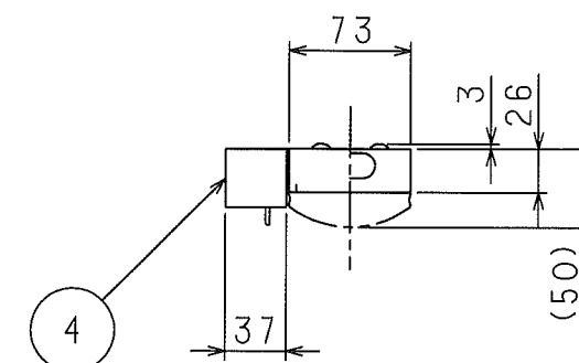
側面詳細図
