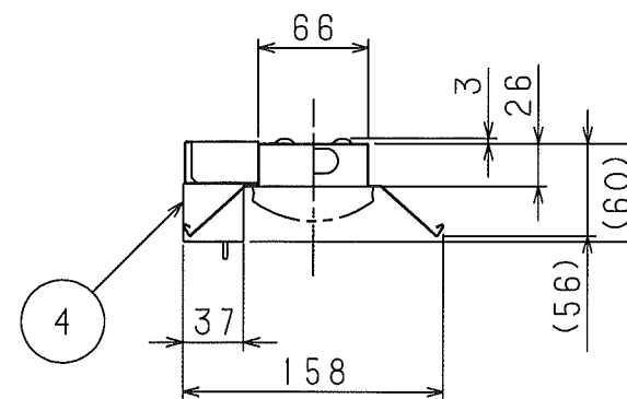
側面詳細図
