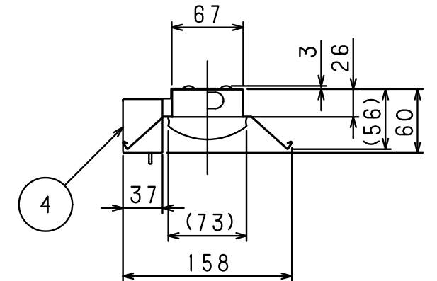
側面詳細図
