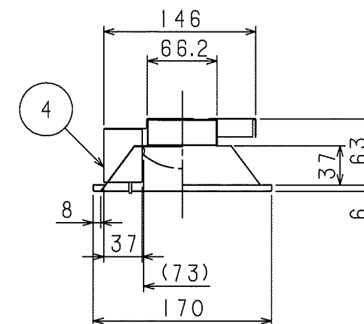
側面詳細図
