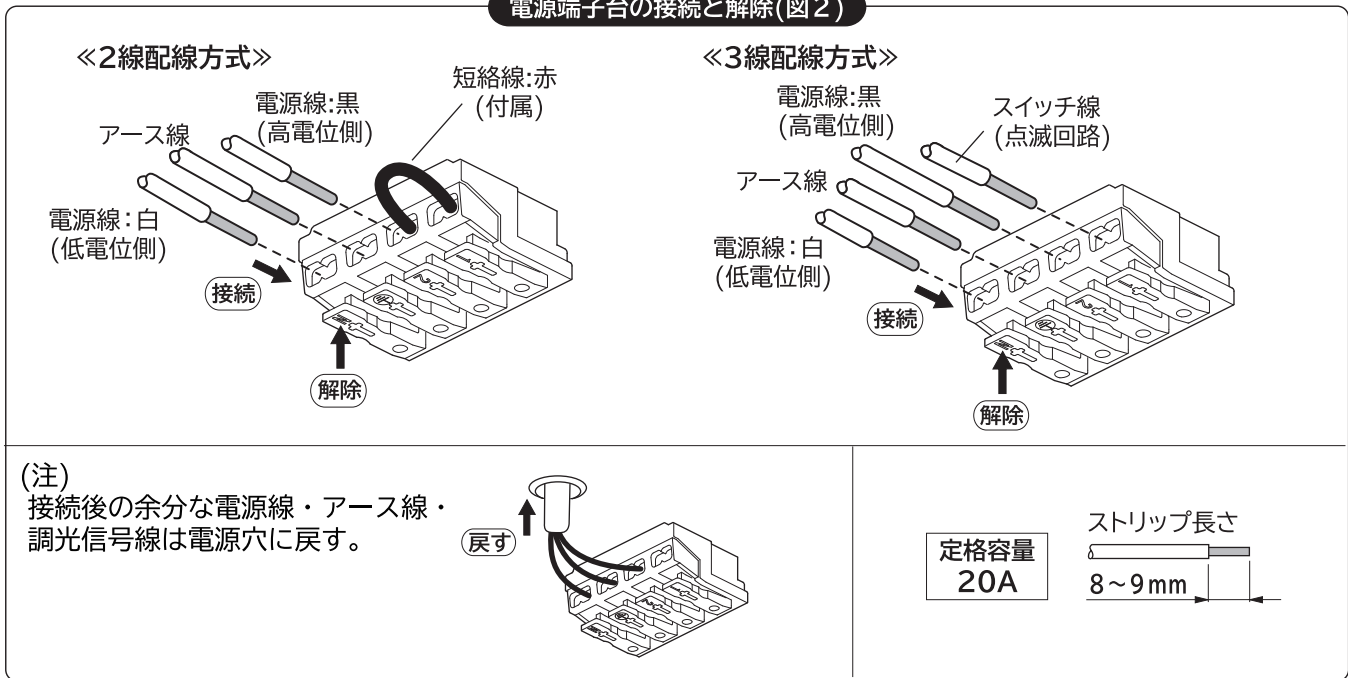
電源端子台の接続と解除(図2)
