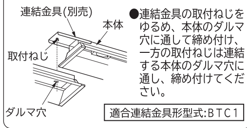
連結のしかた(図1)
