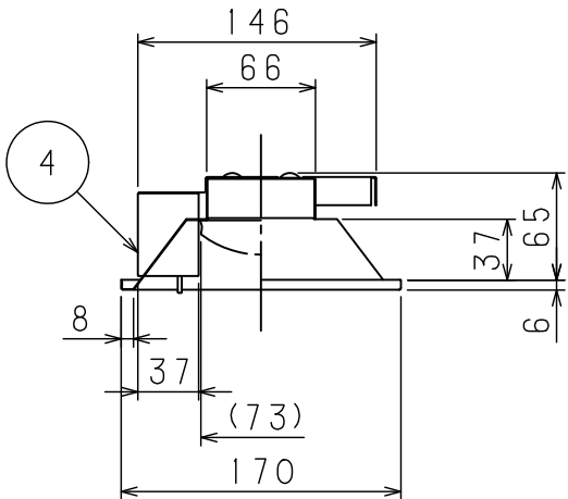
側面詳細図
